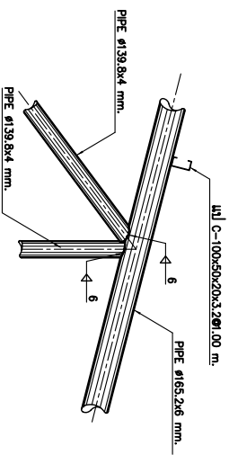
TRS-1 1:20
